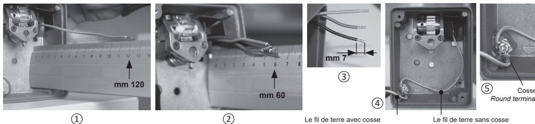
Le fil de terre avec cosse Earth cable with round terminal
